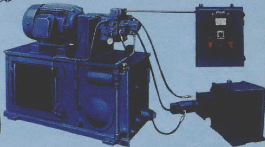
TRANSMISION HIDRAULICA
