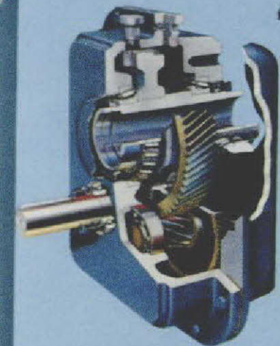
REDUCTOR MONTADO EN EJE
