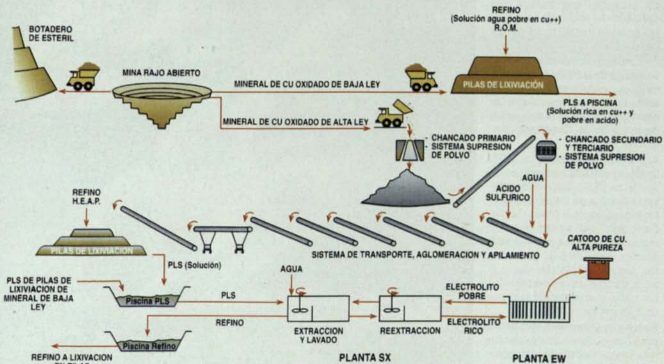
Diagrama general del proceso que se utilizará en el complejo minero Lomas Bayas.
