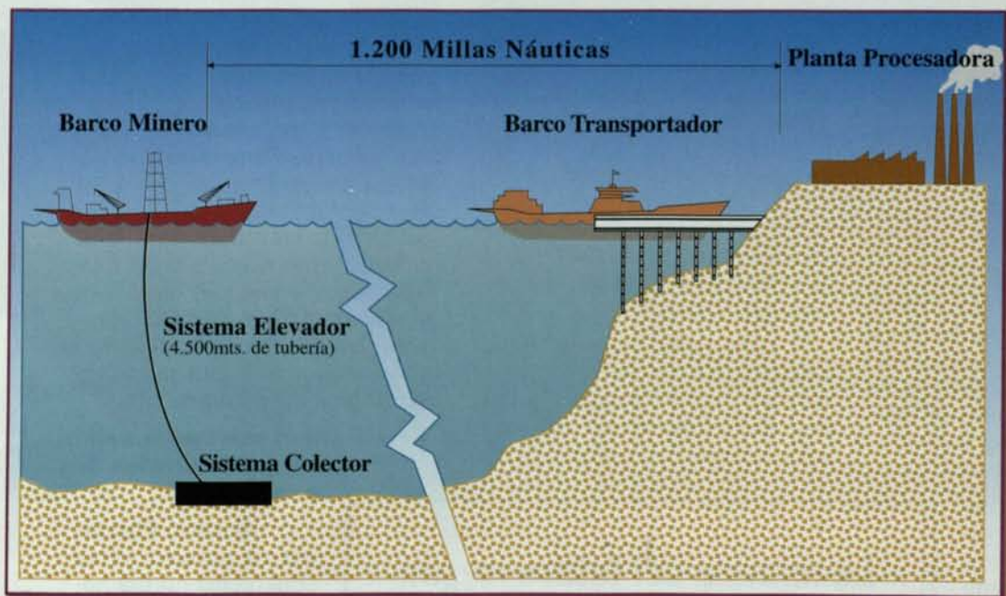
Los componentes básicos de la minería marina son el aparato colector, el sistema elevador, el barco minero y los barcos transportadores. Se estudia también el uso de submarinos dirigidos por control remoto.
