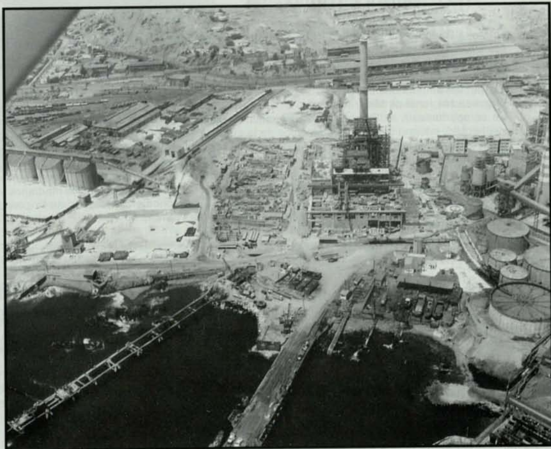
Arriba, la Central termoeléctrica Nueva Tocopilla, ubicada en el Norte Grande, contribuirá al abastecimiento energético de la gran minería. Después, aparece la Central Termoeléctrica Guacolda, en la Tercera Región; al medio, la Planta de Constitución, luego la de Ventanas y la Cuarta Unidad de Piedra de Aguila.
