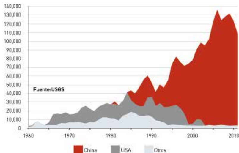
PRODUCCIÓN HISTÓRICA DE TIERRAS RARAS (TON)
