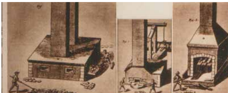
Imágenes de hornos tipo reverbero usados para fundir cobre, a partir del aporte de Lambert.
