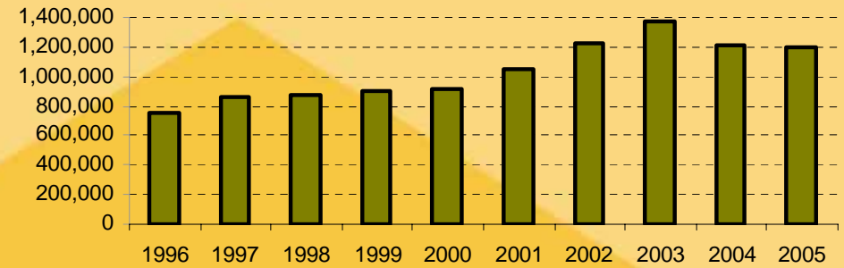
Producción de Zinc, 1996-2005 (TMF)
